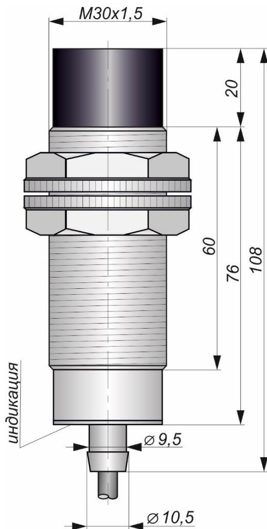
Габаритный чертеж
